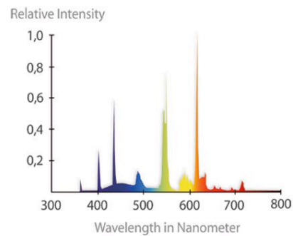
Gewöhnliche Sparlampe 4200° Kelvin - CRI 83
